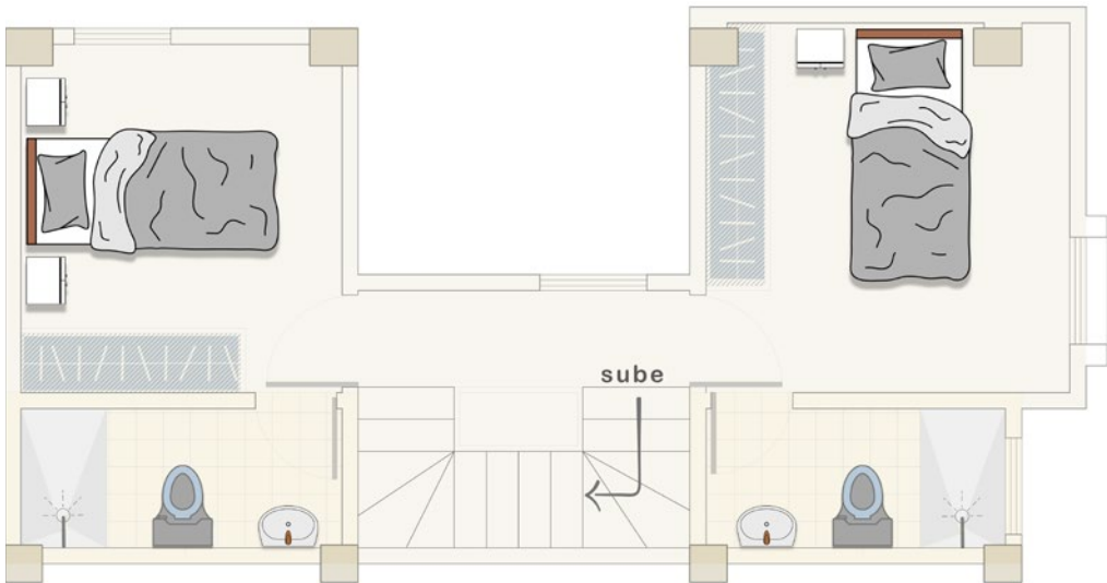
NIVEL + 8.10 PLANTA ALTA Área cubierta casa 4: 43.52m 2
